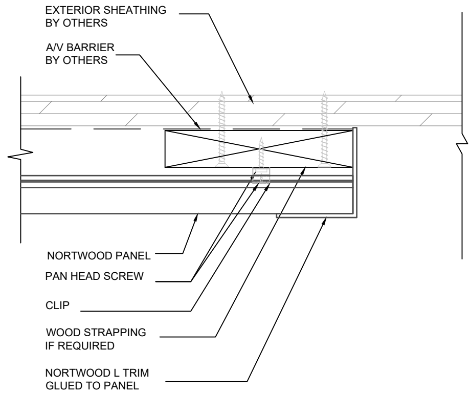
HORIZONTAL START INST. TYP.
